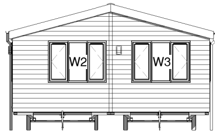
2 Side B 1 : 120
