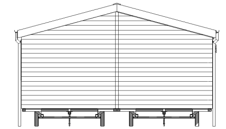
5 Side D 1 : 120
